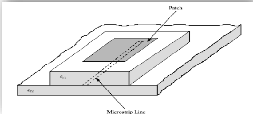
Gambar 3.1 Geometri patch antenna mikrostrip dengan teknik pencatuan electro-magnetically coupled
